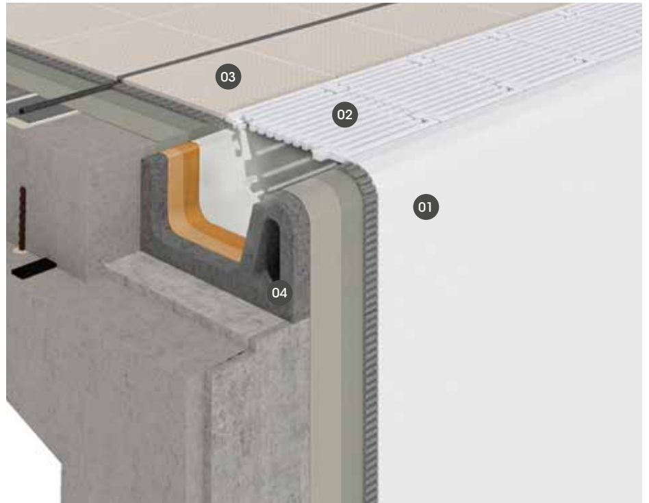
03 240 pastilla Indubeige 24,4 x 24,4 cm Porcelain tile
